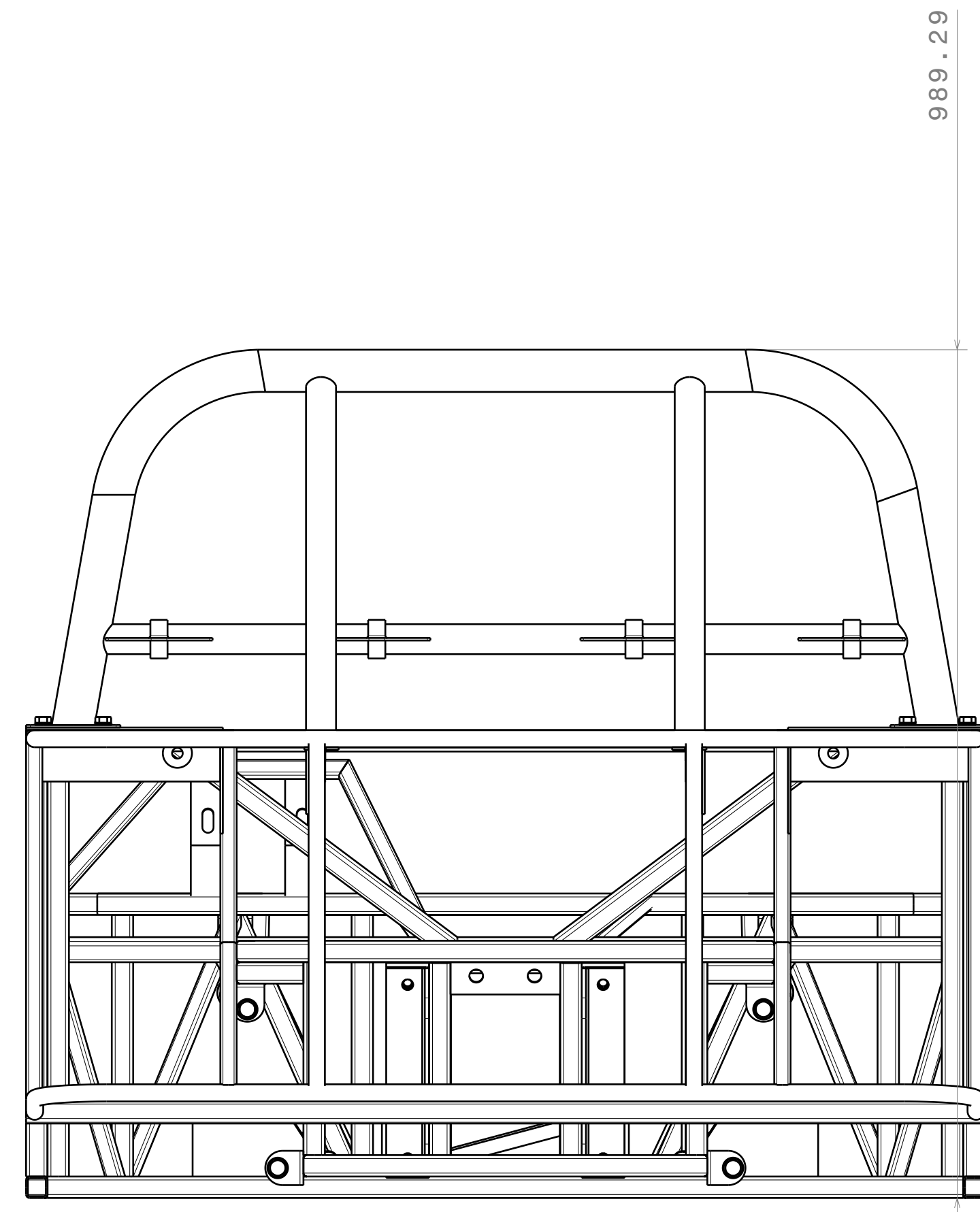
Vue de droite Echelle : 1:6
