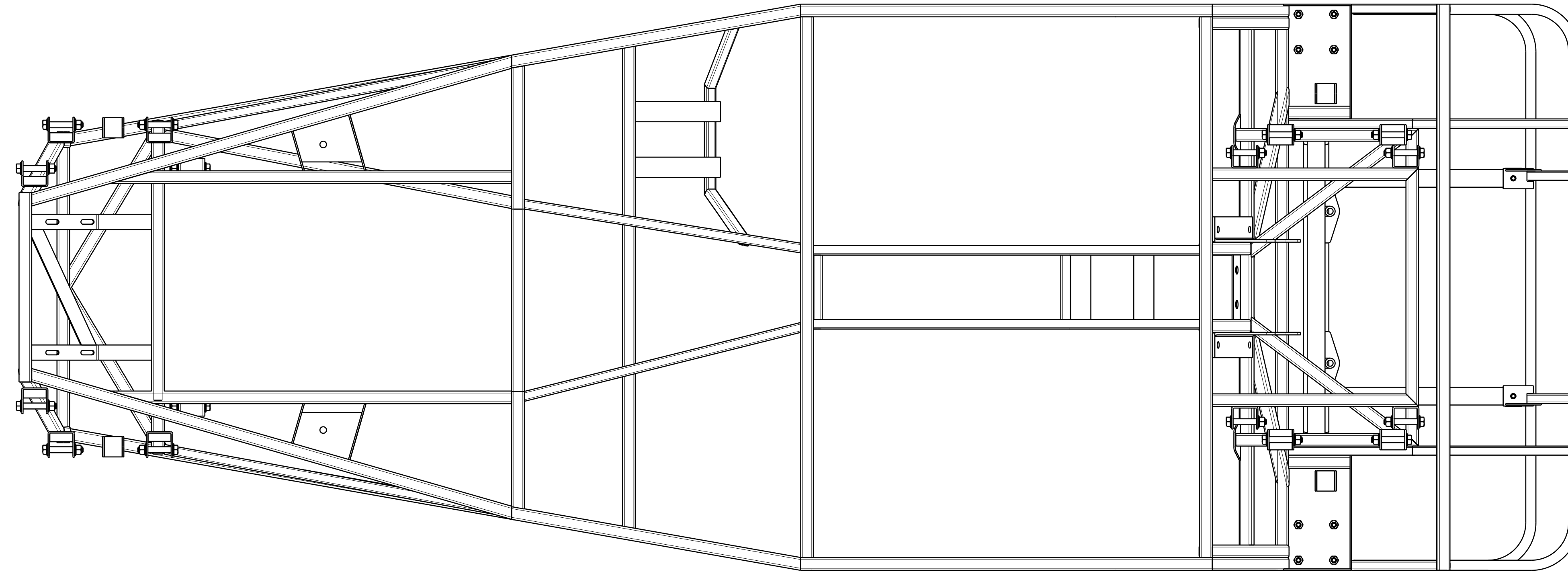
Vue de dessous Echelle : 1:6
