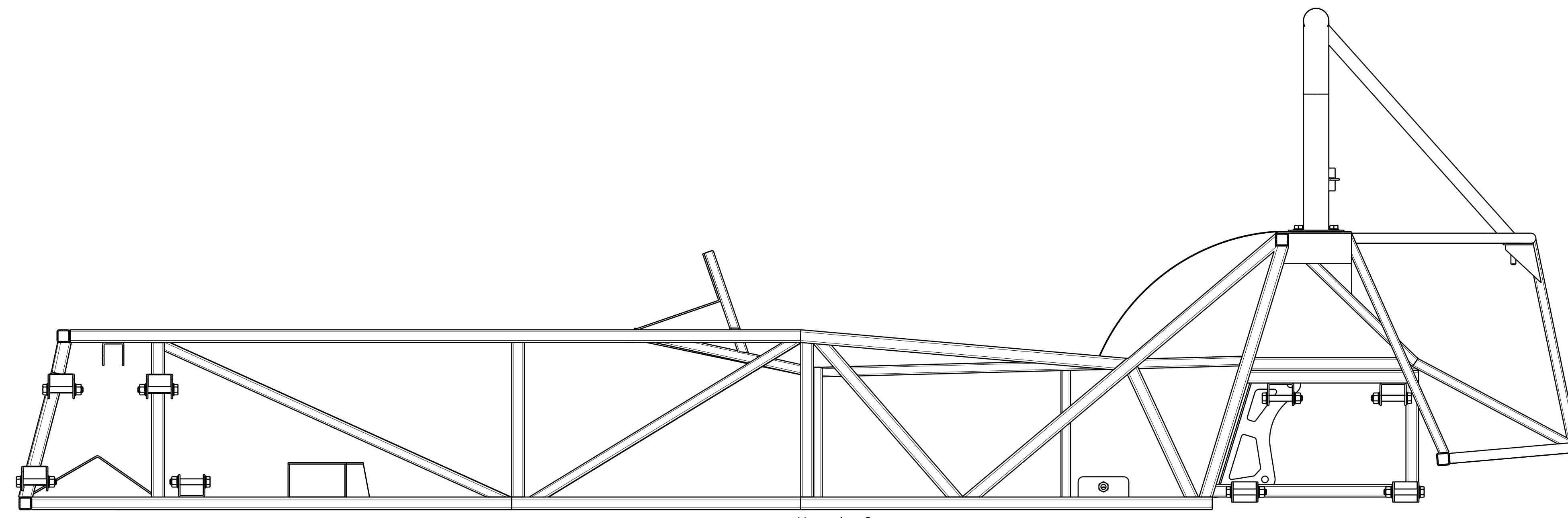
Vue de face Echelle : 1:6
