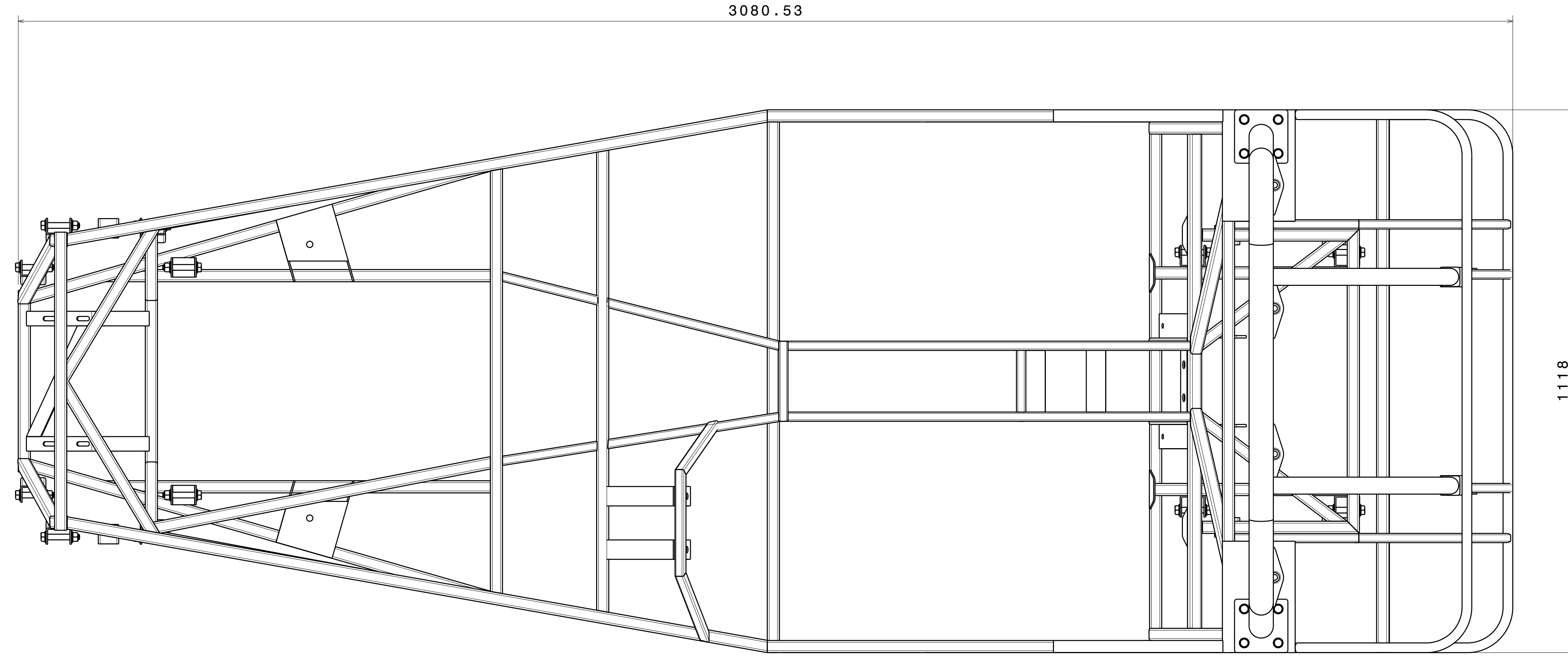
Vue de dessus Echelle : 1:6
