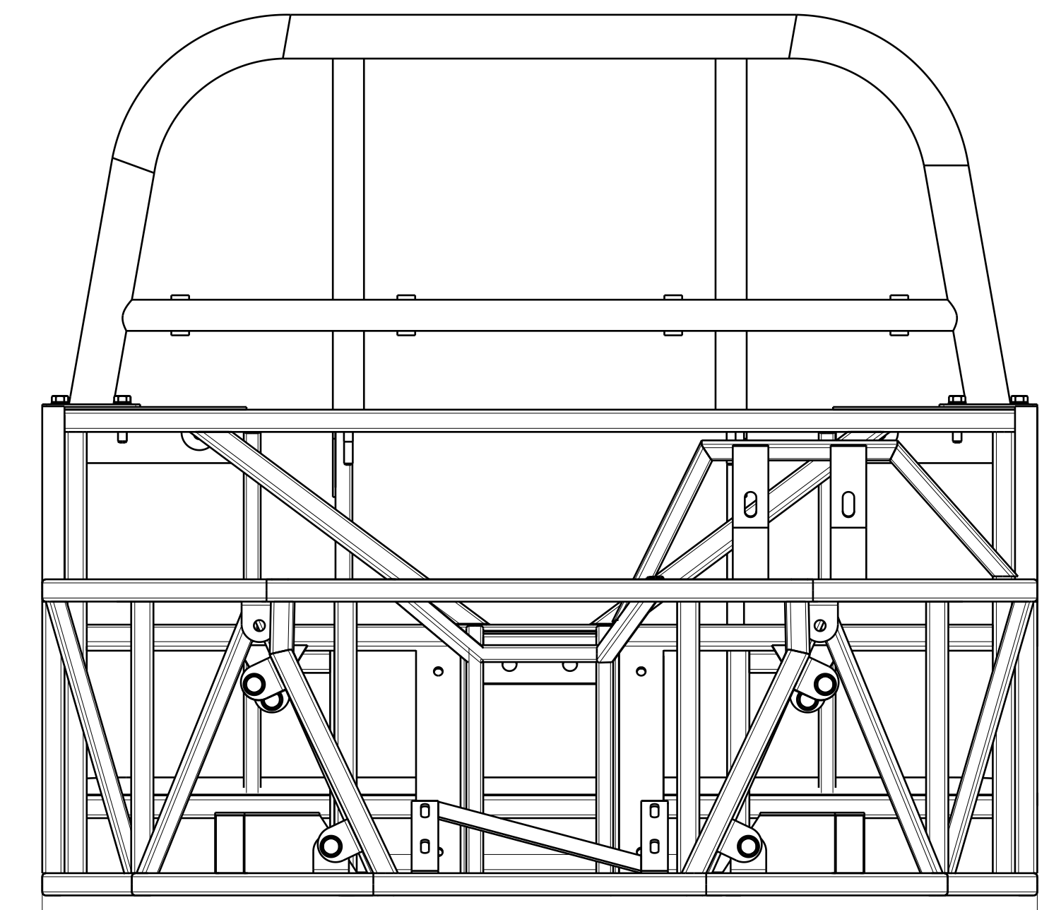
Vue de gauche Echelle : 1:6
