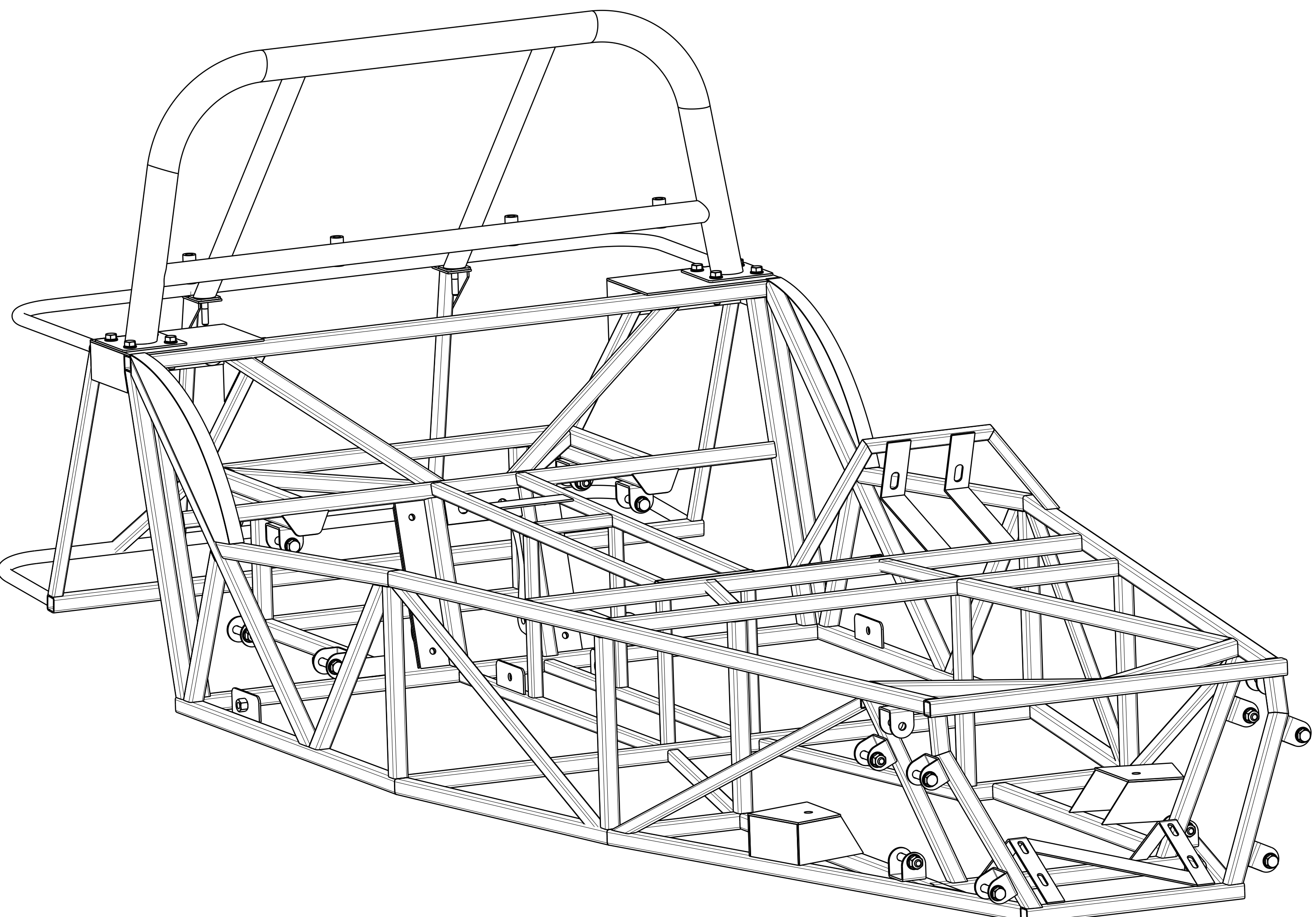
Vue isométrique Echelle : 1:5
